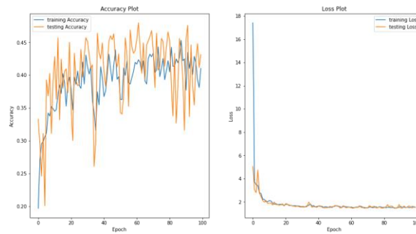
Gambar 7 Grafik Model MLP
