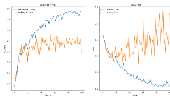
Gambar 6 Grafik Model CNN
